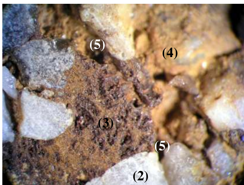
08_3 : Micro conglomérat à ciment ferrugineux (détail de 08_2).
