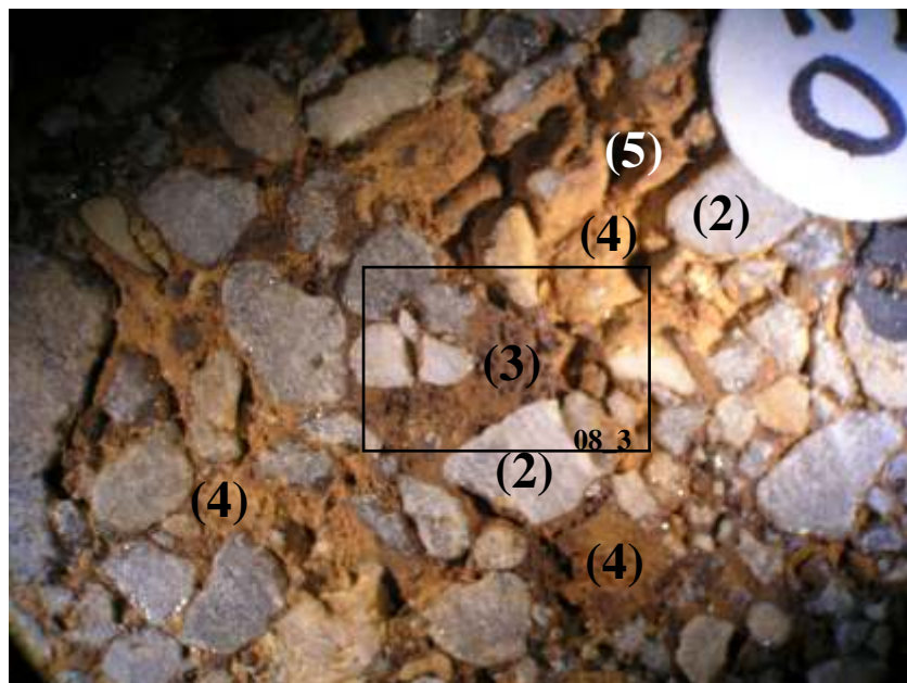
08_2 : Micro conglomérat à ciment ferrugineux (détail de 08_1).
