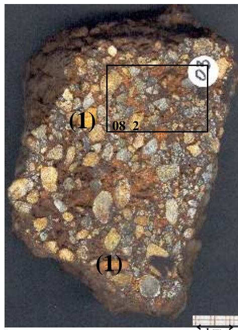
08_1 : Micro conglomérat à ciment ferrugineux. Echelle 1/1.
