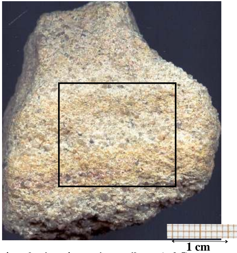
10_1 : Grès arkosique à matrice argileuse (x 2.5)
