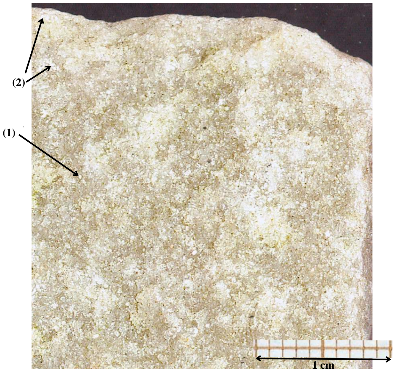
30_2 : Grès quartzite, détail (x 6) de 30_1 : observer les grains sectionné et les grains apparaissant en relief
