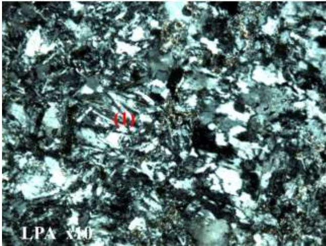
Photo 165 : Détail de la matrice argileuse (1) montrant la disposition en plaquette grise à faible biréfringence de certains minéraux qui pourraient être de la kaolinite.
